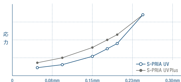
圧縮応力曲線
