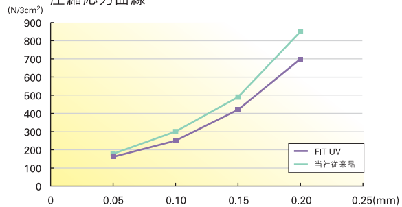
圧縮応力曲線
