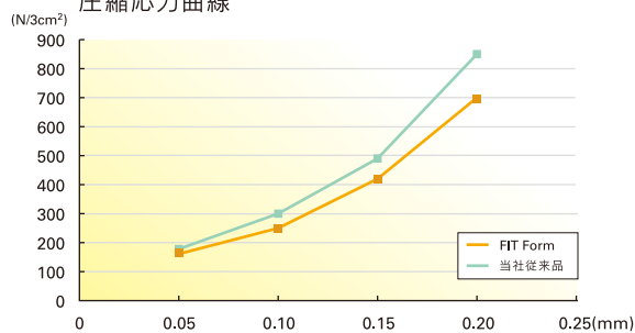
圧縮応力曲線
